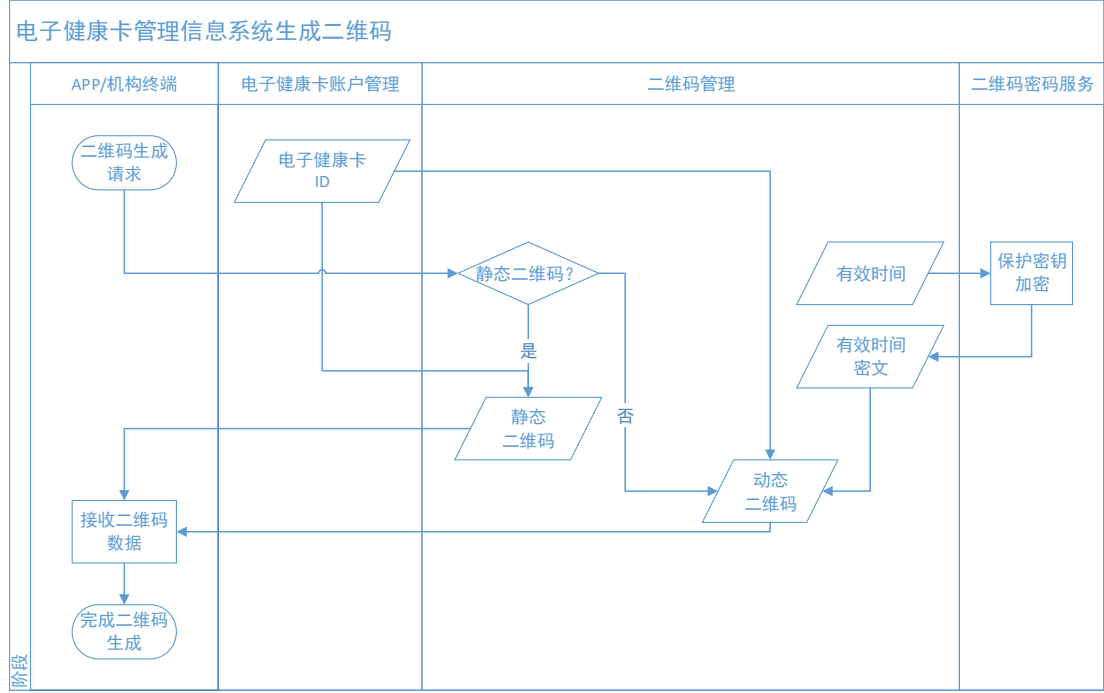
图 6.1 二维码生成流程
