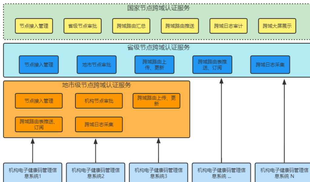
图 2.1 跨域认证服务总体架构图
